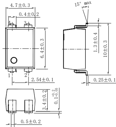
DIP4
